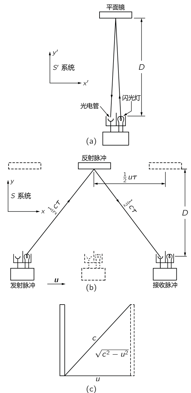
图 15.3: (a) 一个“光钟”静止在 S' 坐标系中；(b) 一个同样的，相对于 S 坐标系运动的钟；(c) 在正在运动的“光钟”中，光束经过的斜向路程示意图
