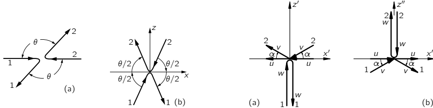
图 16.2: 两个以相等速率、相向运动的相同粒子所发生的弹性碰撞的两种视图
