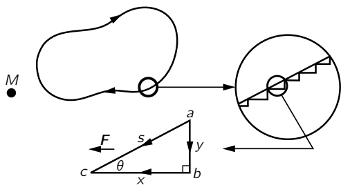
图 13.4: 一条光滑闭合路径，表明用一系列径向与圆周阶梯近似表示的放大大片段和一个阶梯的放大图
